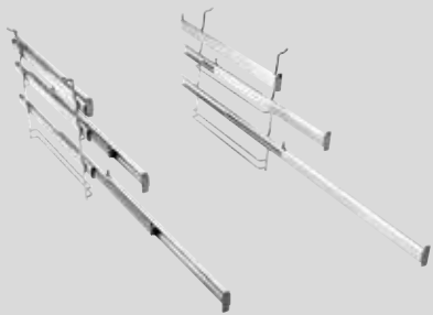
3fach-Vollteleskopauszüge für Superior-Modelle (471093)
